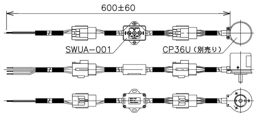
CP36U取付イメージ (尺度1:4)
